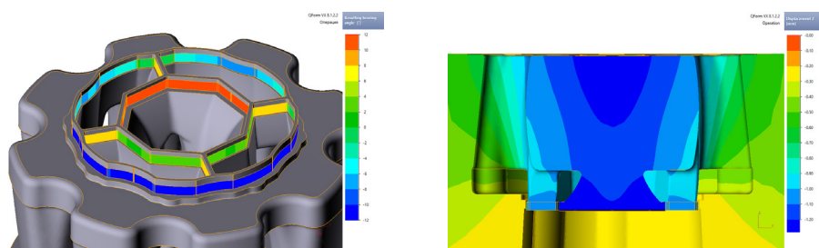
Анализ напряжений и деформаций в инструменте
